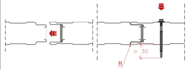
Detalle de Encaje - Joint Detail
