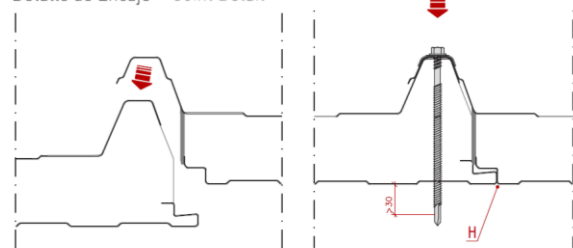
Detalle de Encaje - Joint Detail
